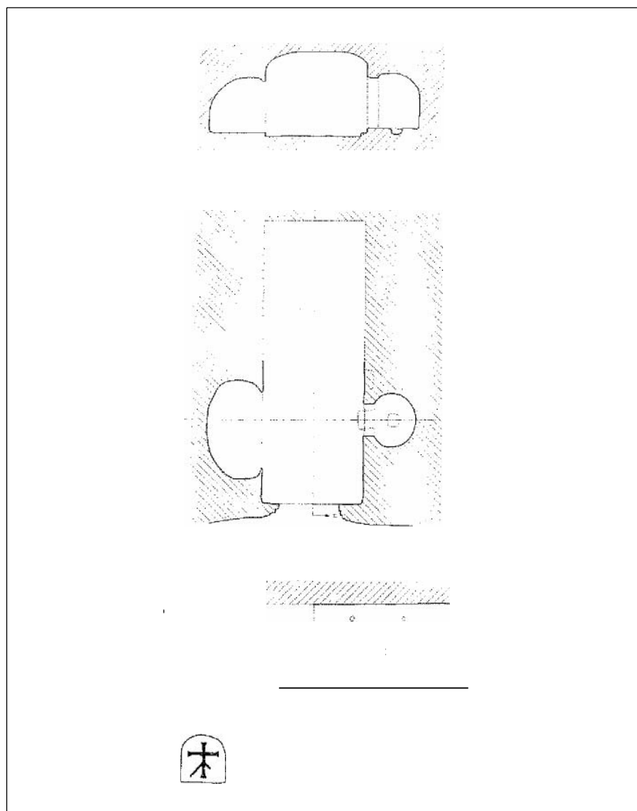
Cueva 2. Iglesia. Sección trantsversal hacia li cabecera.
